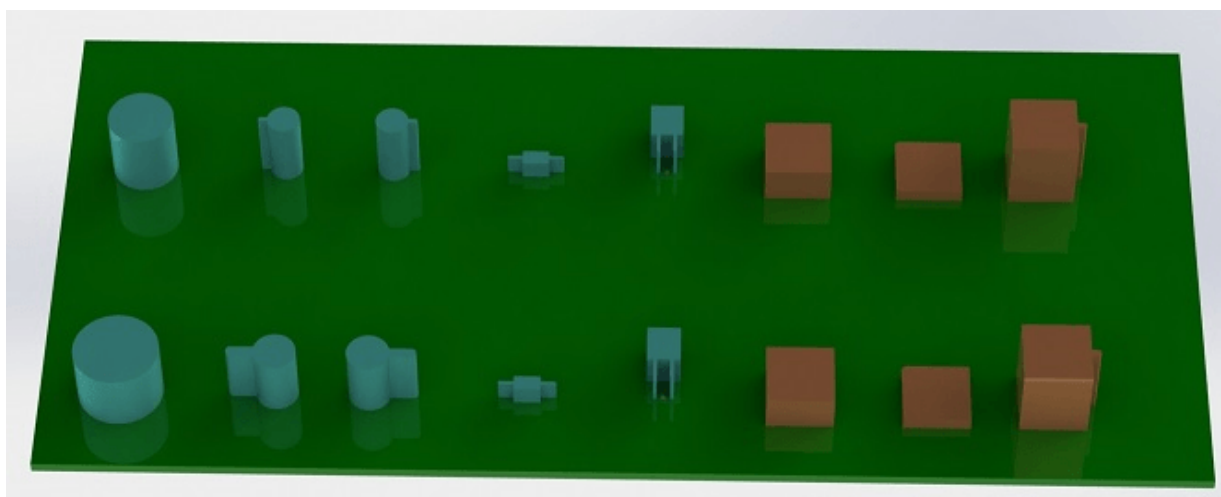
Rysunek 4: Próbkę konturów generowane przez programy idfrect oraz idfcyl zrenderowane przez SolidWorks.
